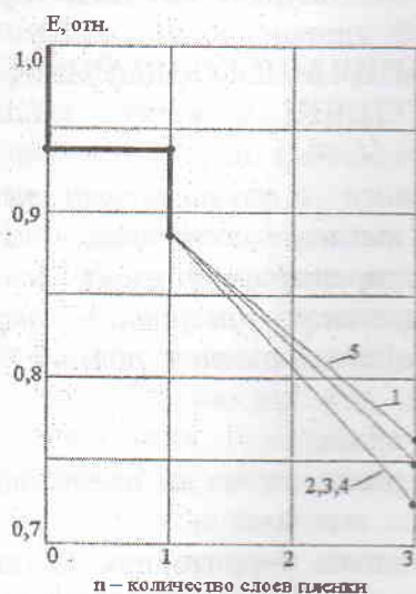
Рис. 1. Изменение светопропускания многослойной прозрачной изоляции гелиотеплиц в зависимости от количества слоев в ясный день с первым стеклянным слоем. Полиэтиленовые пленки толщиной: 1 – 0,024 мм; 2 – 0,04 мм; 3 – 0,08 мм; 4 – 0,18 мм; 5 – 0,32 мм.
