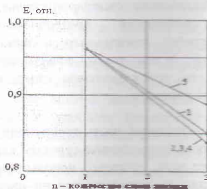
Рис. 1. Изменение светопропускания многослойной прозрачной изоляции гелиотеплиц в зависимости от количества слоев в ясный день с первым стеклянным слоем. Полиэтиленовые пленки толщиной: 1 – 0,024 мм; 2 – 0,04 мм; 3 – 0,08 мм; 4 – 0,18 мм; 5 – 0,32 мм.
