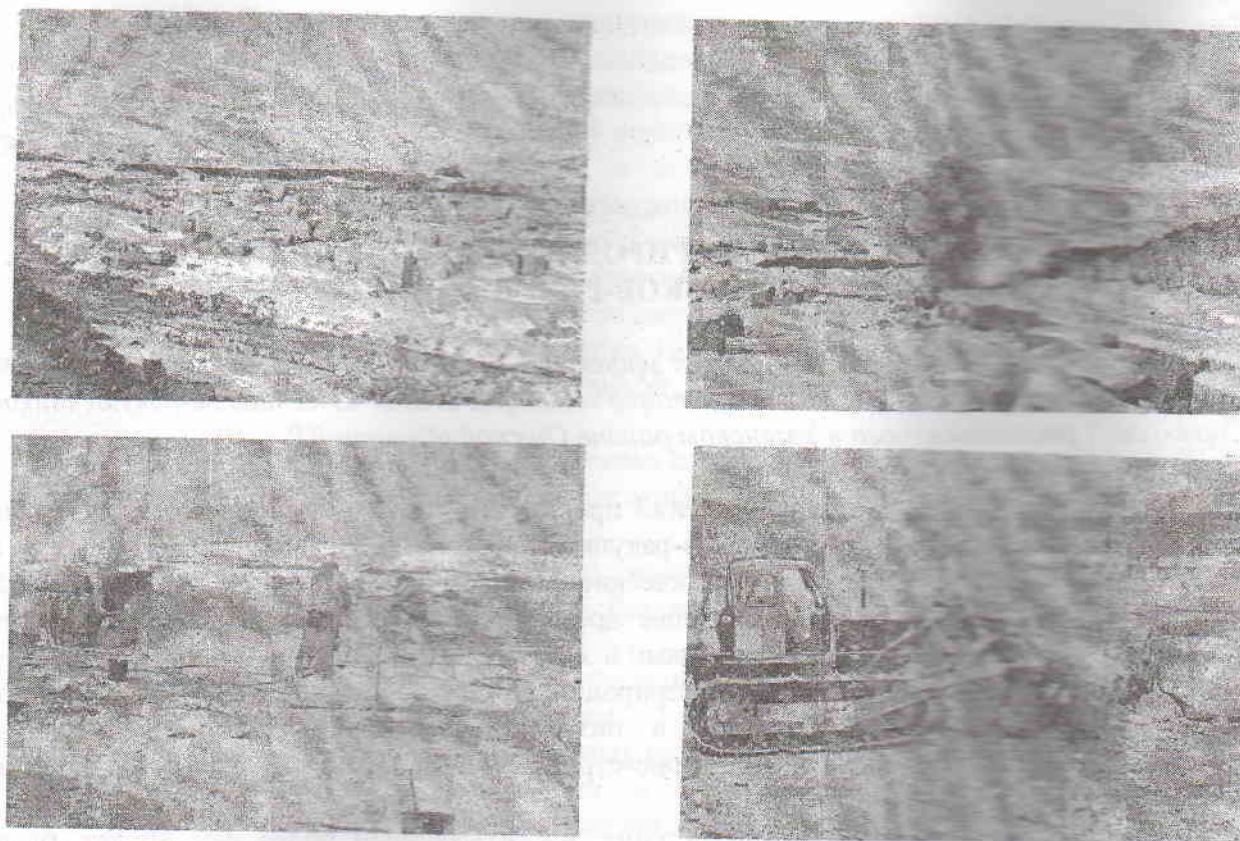
Рис. 1. Технология добычи блоков буровзрывным способом на карьере известняка-ракушечника «Сары-Таш» до середины 1990-х годов
