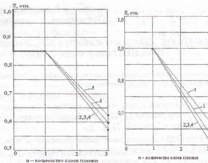
Рис. 3. Изменение светопропускания многослойной прозрачной изоляции гелиотеплицы в зависимости от количества слоев в пасмурный день с первым стеклянным слоем. Полиэтиленовые пленки толщинами: 1 – 0,024 мм; 2 – 0,04 мм; 3 – 0,08 мм; 4 – 0,18 мм; 5 – 0,32 мм.
