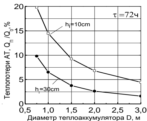
Рисунок 4 - Влияние объема (диаметра) аккумулятора тепла на её тепловые потери при толщине теплоизоляции 10 см и 30 см и времени хранения 72 часа
