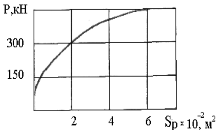
Рисунок 2- Диаграмма изменения усилия раскола в зависимости от площади раскола [1]
