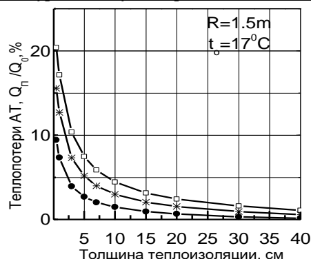
Рисунок 3 - Тепловые потери водяного двухслойного шарового аккумулятора тепла с радиусом 1.5м, в зависимости от толщины теплоизоляции при различных сроках хранения воды: 24ч - •, 48ч - ×, 72ч - □.
