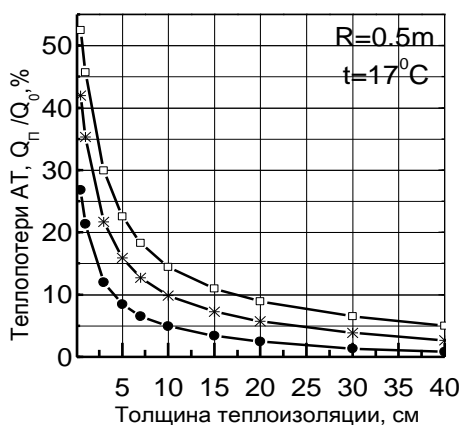
Рисунок 2 - Тепловые потери водяного двухслойного шарового аккумулятора тепла с радиусом 0.5 м, в зависимости от толщины теплоизоляции при различных сроках хранения воды:
