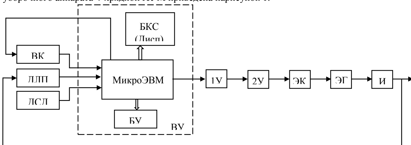
Рисунок 1- Структурная схема системы контроля и регулирования одной рабочей щели уборочного аппарата ХУМ.
