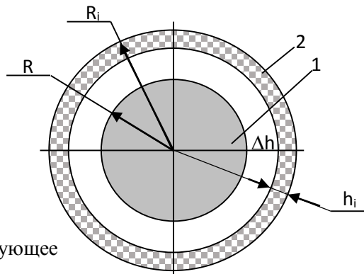
Рисунок 1 - Схема двухслойного шарового аккумулятора тепла
