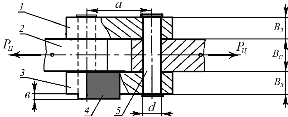
1,3 – боковые звенья; 2 – среднее соединяющее звено; 4 – твердосплавный резец; 5 – ось. Рисунок 2 - К определению условий динамической прочности звеньев режущей цепи
