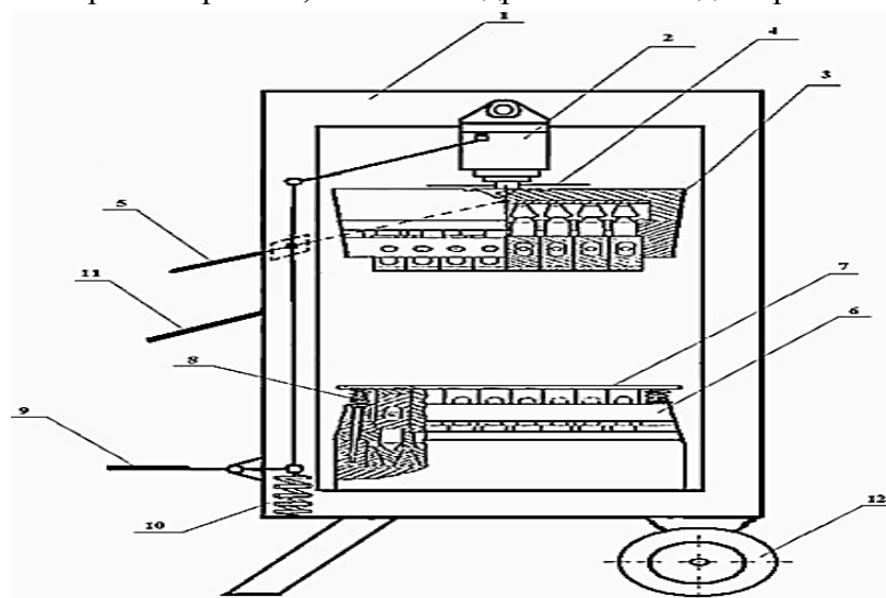
Рисунок 3- Конструкция переносного камнекольного пресса ПКП-300
