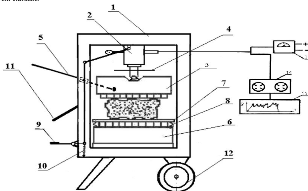
Рисунок 1- Конструктивная схема переносного камнекольного пресса ПКП-300:
