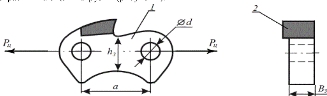
1 - звено режущей цепи; 2 – твердосплавный резец. Рисунок 1 - Режущее звено цепного рабочего органа
