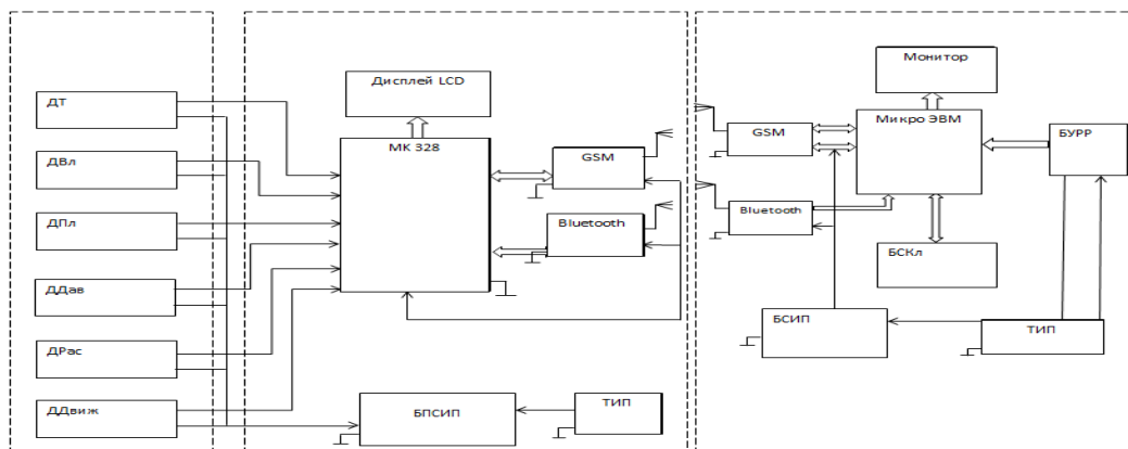
Рисунок 1- Структурная схема системы мониторинга пожарной безопасности состояния объектов
