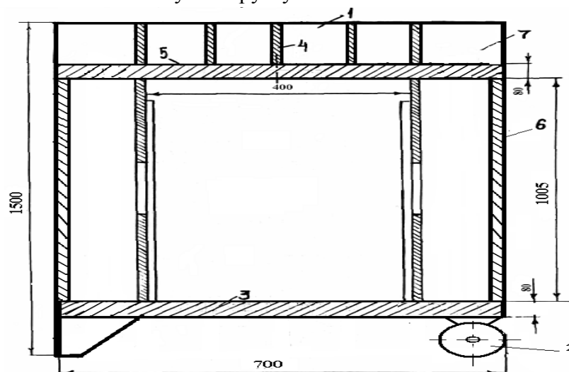
Рисунок 4 - Конструктивная схема станины переносного камнекольного пресса ПКП-300
