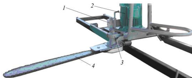
Камнерезные машины с цепными рабочими органами КМЦ-1 и КМЦ-2 (2015 г.) Авторы: М.Т. Мамасаидов, М.М. Исманов
